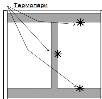
Рисунок 3 – Схема розміщення термопар на зразках сталевій колони з коробчастим перерізом
