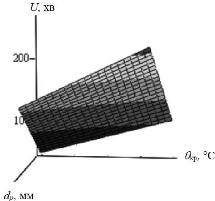
Рисунок 9 – Поверхня залежності часу досягнення критичної температури від обраних параметрів вогнезахищеного елемента сталевій конструкції
